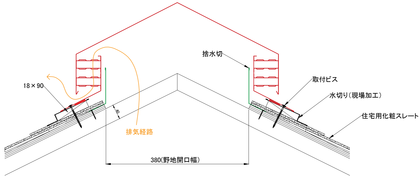
隅棟部を棟包納めの場合
